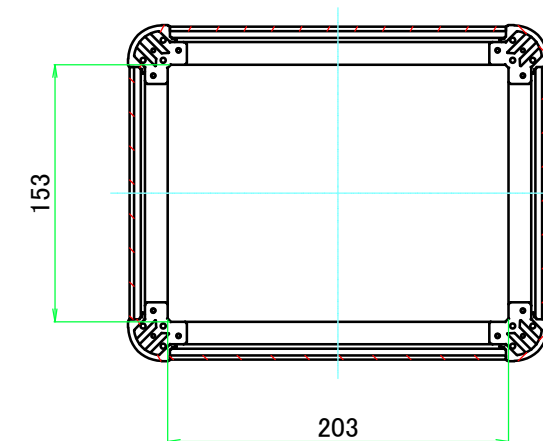
C-C ( 1 : 4.5 )
