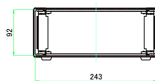
B-B ( 1 : 4.5 )
